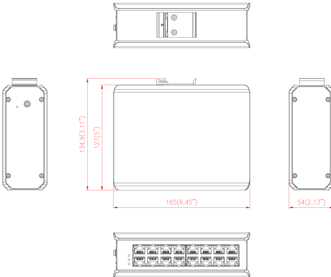
尺寸图
