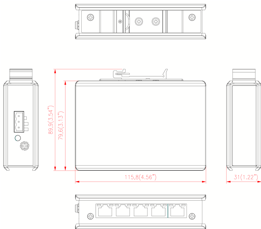
尺寸图
