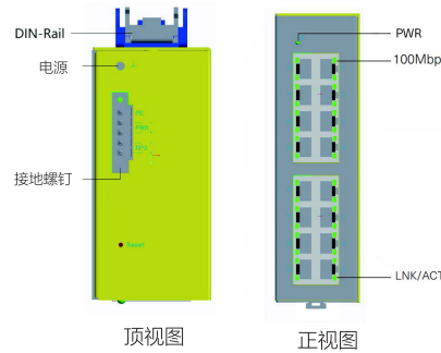
顶视图
