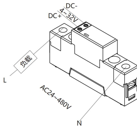
接线图 Wiring Diagram
