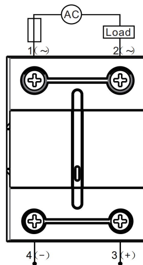
接线图 Wiring Diagram
